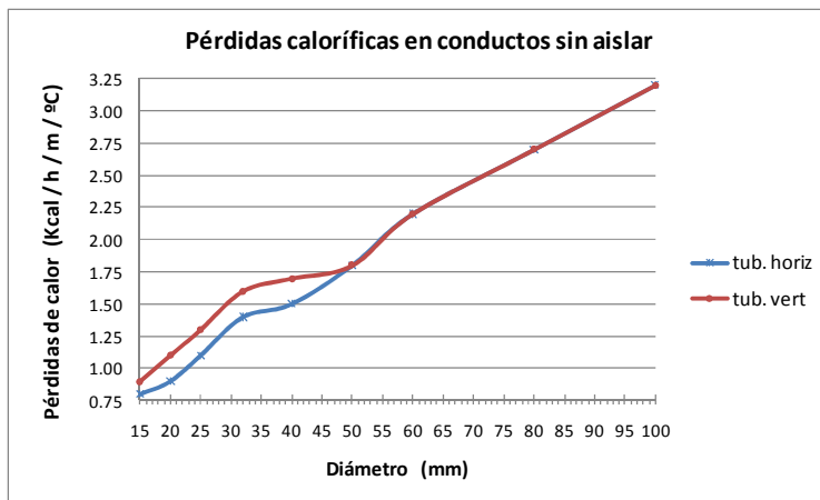
Figura 16.5. Pérdidas de calor en conductos sin aislar
