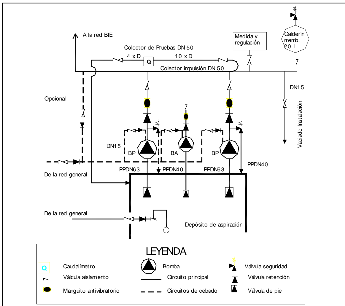
Figura 16.9. Ejemplo de instalación de sistema contra incendios con 2 bombas principales eléctricas y bomba auxiliar, más grupo electrógeno.
