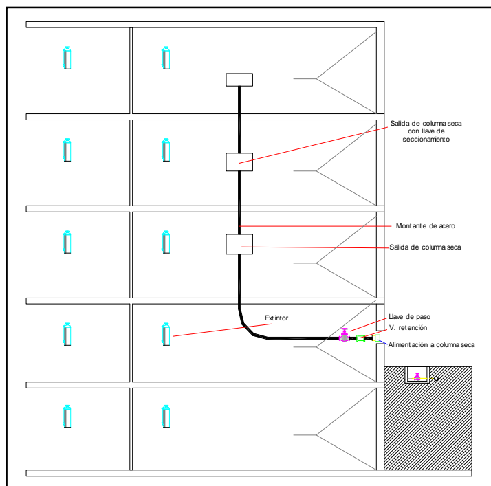
Figura 16.6. Instalación de columna seca
