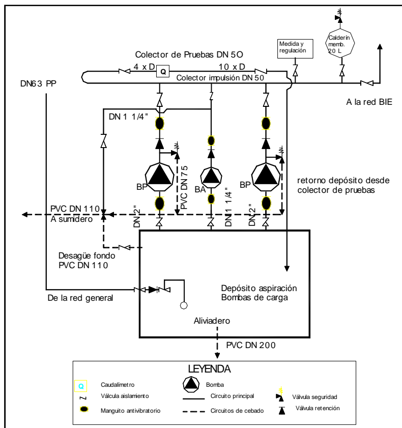
Figura 16.10. Ejemplo de instalación de sistema de bombeo para bocas de incendio equipadas.
