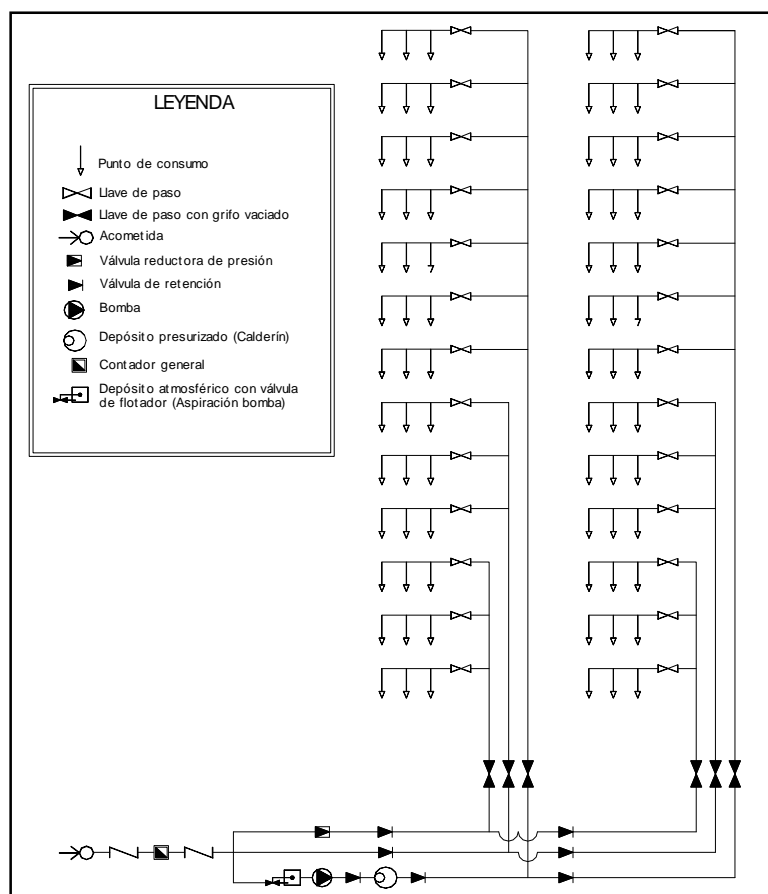
Figura 16.2. Instalación con contador único y varias columnas montantes
