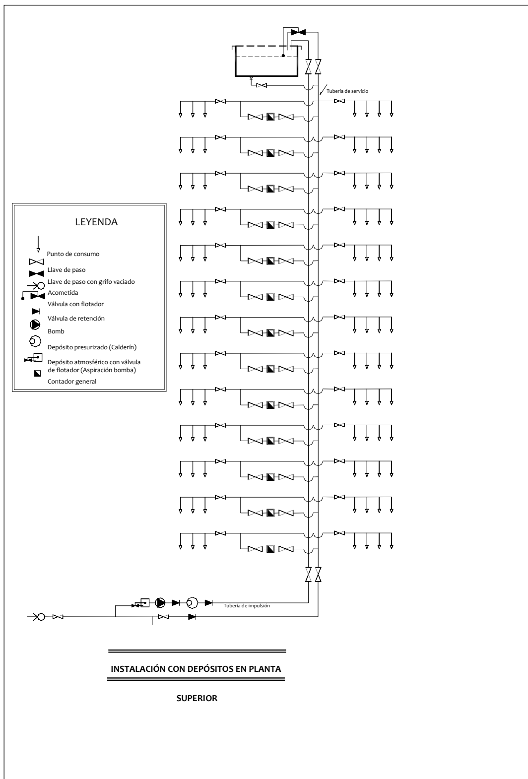
Figura 16.3. Suministro con depósito superior y contador divisionario por planta
