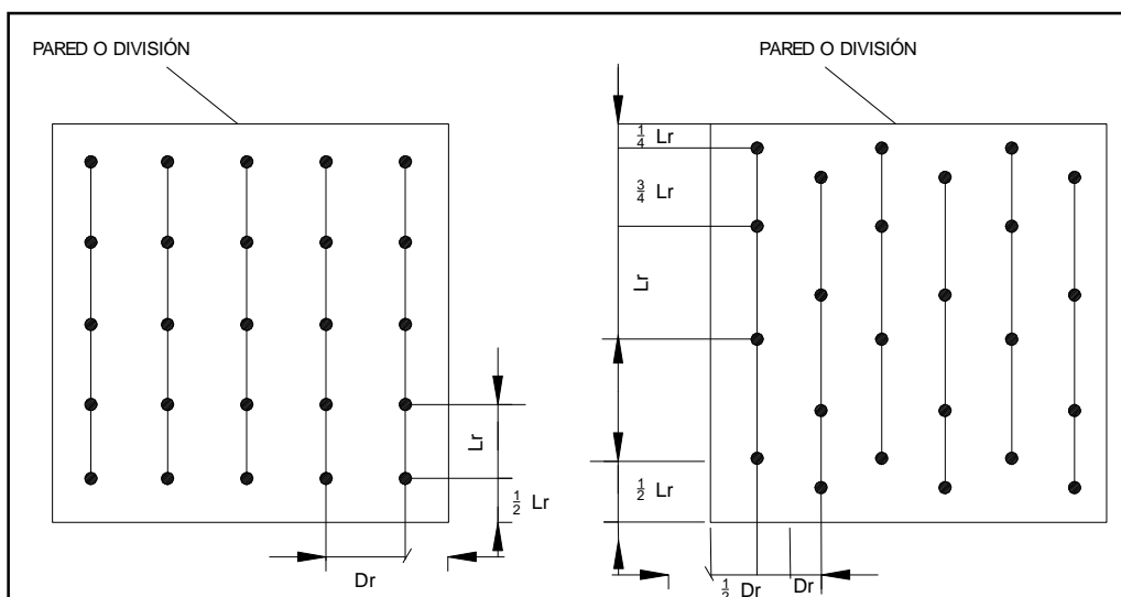
Figura 16.8. Distribución de rociadores
