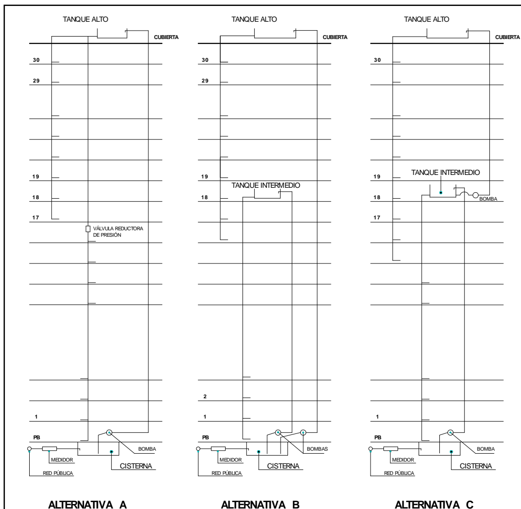
Figura 16.4. Distribución esquemática para edificaciones altas
