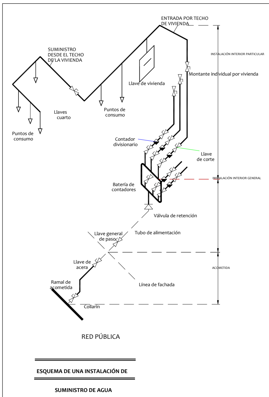
Figura 16.1. Instalación de suministro de agua con batería de contadores
