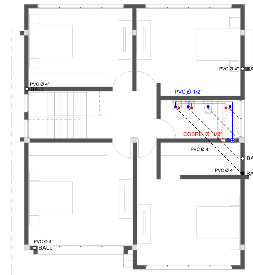
PLANTA ALTA
