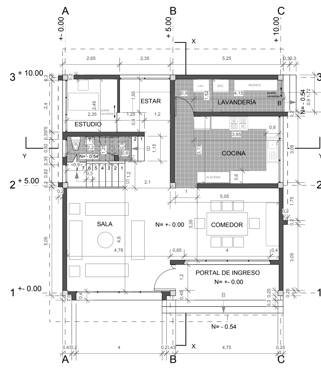
PLANTA BAJA
