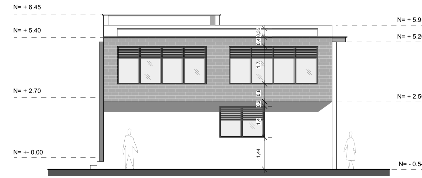
ALZADO POSTERIOR
