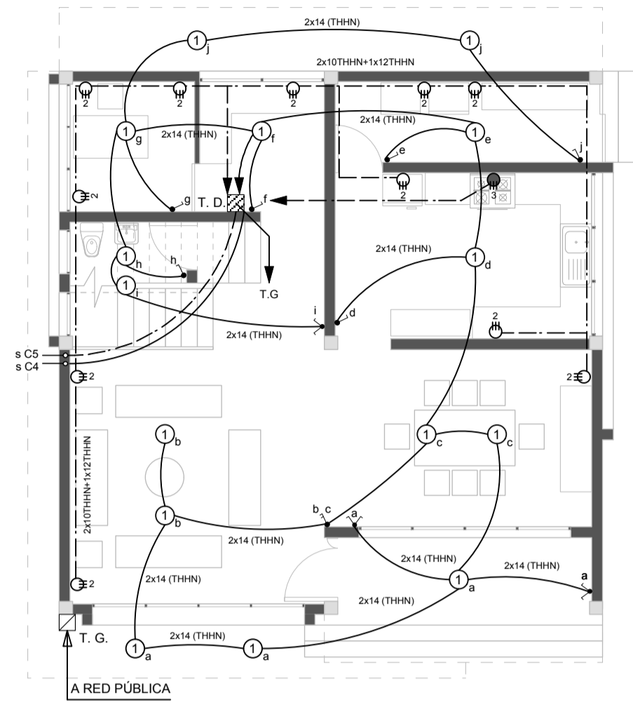
PLANTA BAJA
