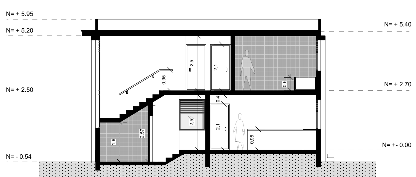
SECCIÓN Y - Y
