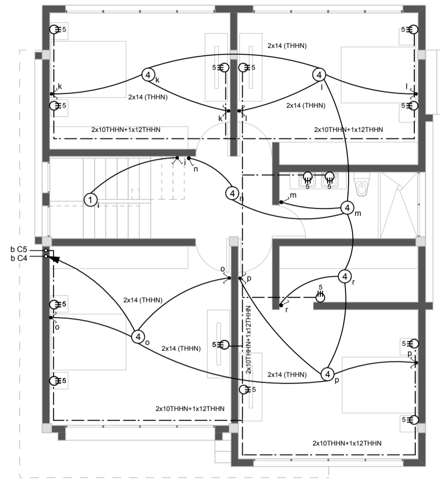
PLANTA ALTA
