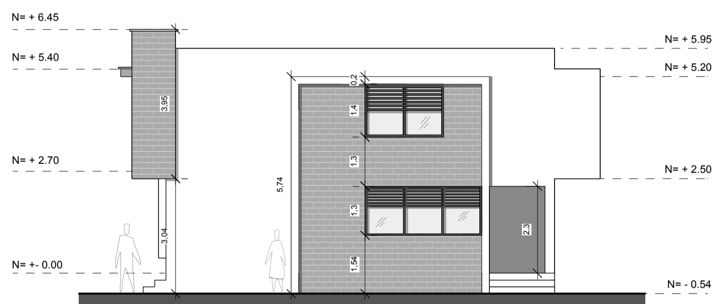
ALZADO LATERAL DERECHO
