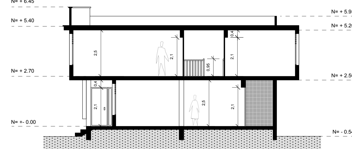
SECCIÓN X - X
