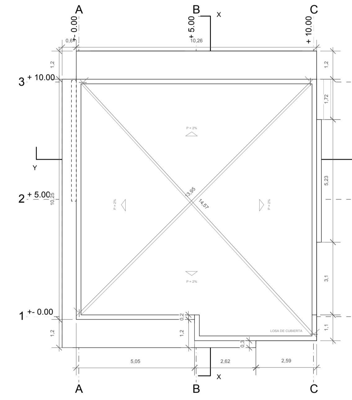
PLANTA DE LOSA
