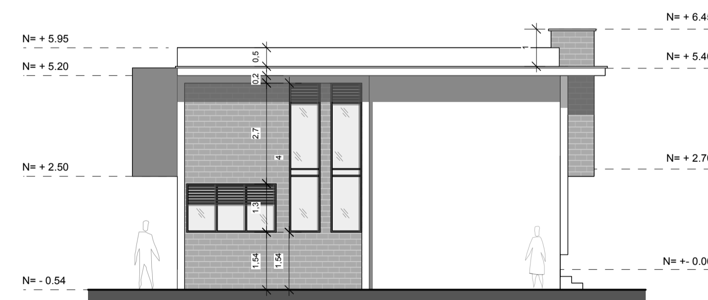
ALZADO LATERAL IZQUIERDO
