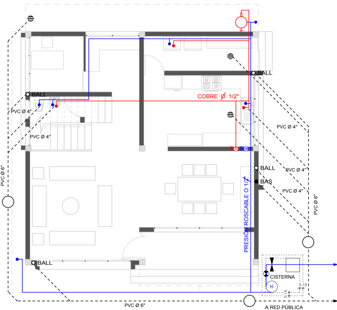
PLANTA BAJA
