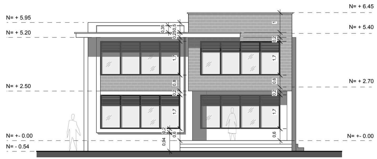
ALZADO FRONTAL
